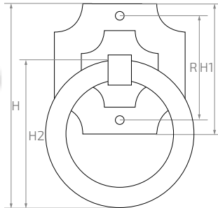
Kołatka Knocker | Geschmiedeter Türgriff
