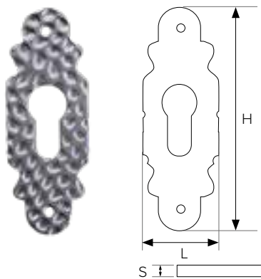
Szyld ozdobny Decorative shield | Dekoratives Schild
