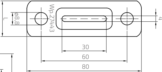
Łącznik przęśta ogrodzeniowego – do przykręcenia Mounting bracket | Montagehalterung
