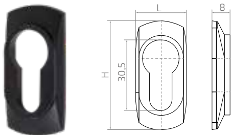
Maskownica wkładki zamkowej YALE YALE lock cylinder bezel | YALE-Schließzylinderblende
