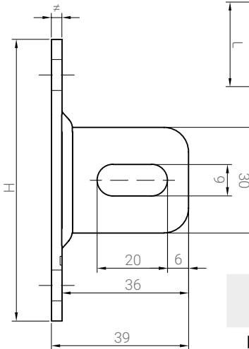
Łącznik przęśta ogrodzeniowego – do przykręcenia Mounting bracket | Montagehalterung
