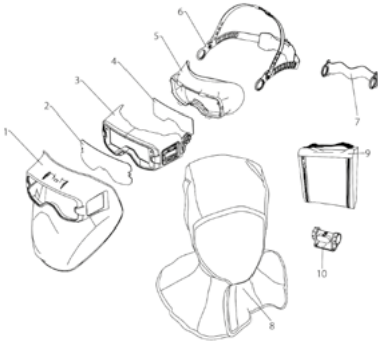
Gogle spawalnicze Star Wire PRO z systemem ADF TRUE COLOR TECHNOLOGY Star Wire PRO welding goggles with ADF TRUE COLOR TECHNOLOGY system | Star Wire PRO Schweißerschutzbrille mit ADF TRUE COLOR TECHNOLOGY System
