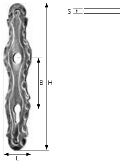
Szyld ozdobny Decorative shield | Dekoratives Schild
