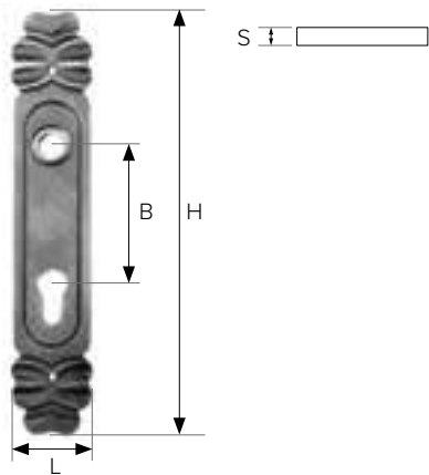
Szyld ozdobny Decorative shield | Dekoratives Schild
