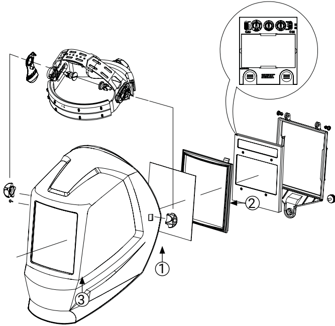
Przyłbica automatyczna Star Wire PRO z systemem ADF TRUE COLOR TECHNOLOGY Star Wire PRO automatic visor with ADF TRUE COLOR TECHNOLOGY system | Star Wire PRO Automatikvisier mit ADF TRUE COLOR TECHNOLOGY System
