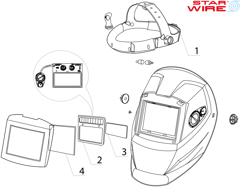
Przyłbica automatyczna Star Wire z systemem ADF Automatic welding helmet Star Wire with ADF filter | Automatic Schweißhelm Star Wirev mit ADF Filter
