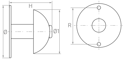
Gałka Knob | Knopf
