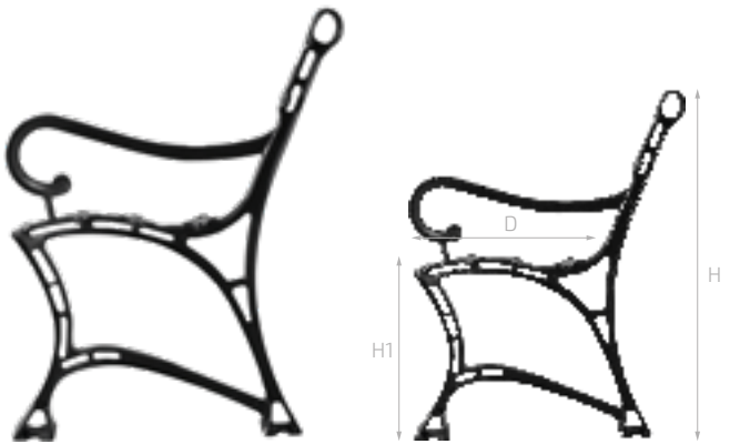
Noga aluminiowa ławki, królewska z podłokietnikiem Aluminium bench leg, royal with armrest | Aluminium-Bankfuß, Royal mit Armlehne
