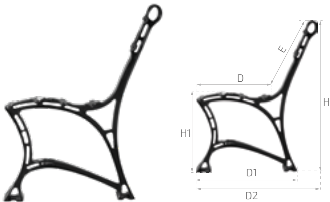
Noga aluminiowa ławki, królewska bez podłokietnika Aluminium bench leg, royal without armrest | Aluminium-Bankfuß, Royal ohne Armlehne
