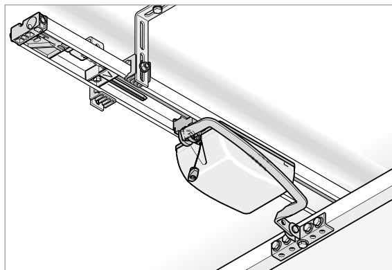
Арт. 3122 Кронштейн для низкой притолоки
