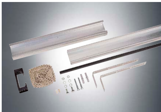
Арт. S10868 ход 543 мм Удлинитель направляющей для привода секционных ворот pro+.
